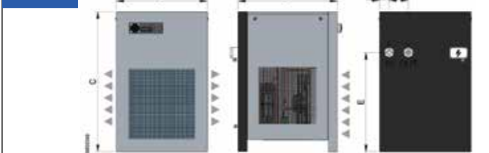
PCD210
